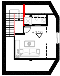
livello sottotetto + 3,50
